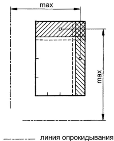
Рисунок 4 – Номинальная нагрузка – оборудование
