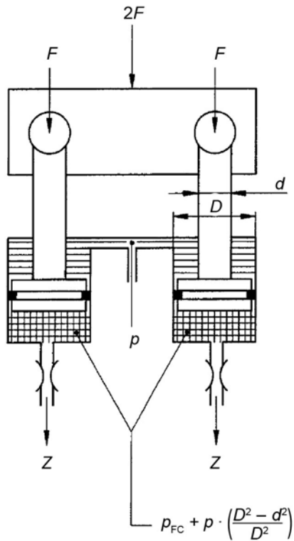
Рисунок 14 – Два цилиндра, работающие на сжатие; обычная работа
