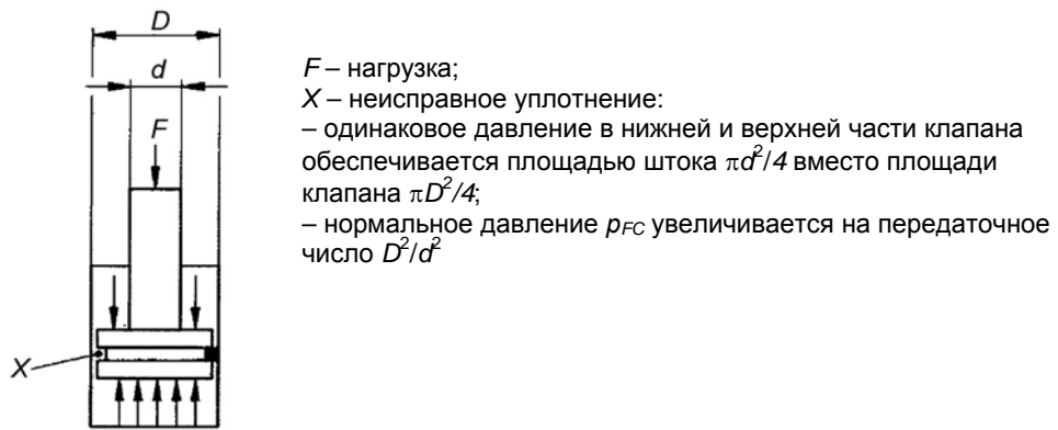
Рисунок 13 – Давление в цилиндре; разгерметизация
