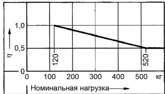
Рисунок 9 – Коэффициент диапазона нагрузки \eta
