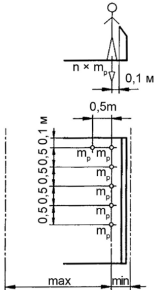
Рисунок 3 – Номинальная нагрузка – персонал
